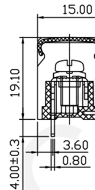
SECTION A-A
