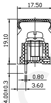
SECTION A-A
