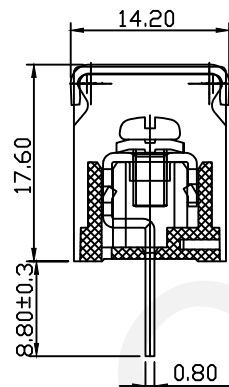
SECTION A-A
