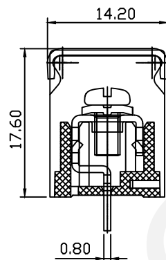
SECTION A-A
