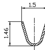
Section:A-A
