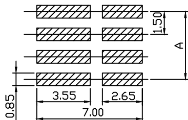
P.C.Board Layout
