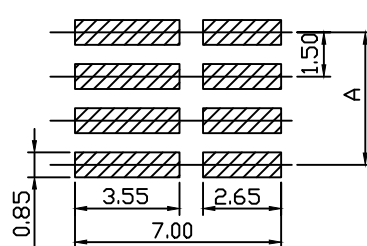
P.C.Board Layout
