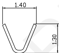
B-B
